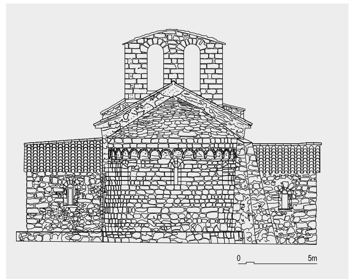
Alzado este
