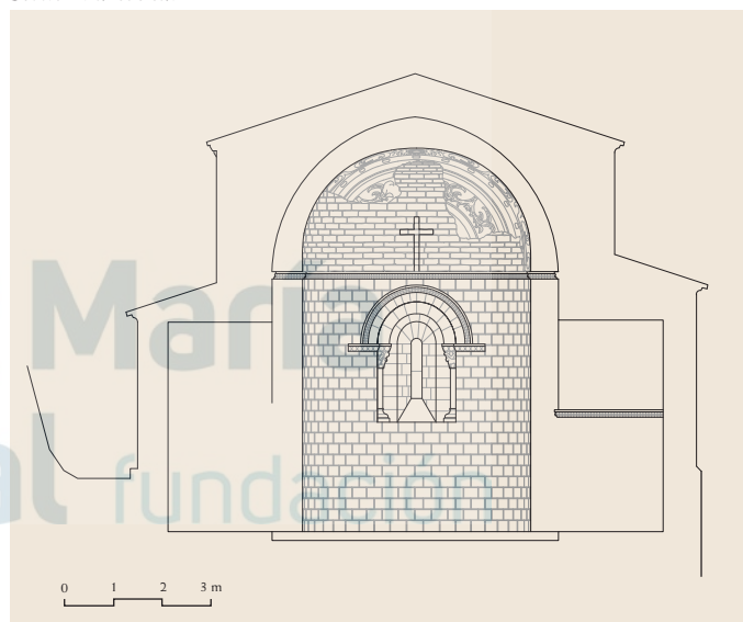
Sección transversal
