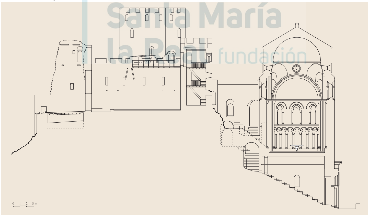
Sección transversal de la iglesia
