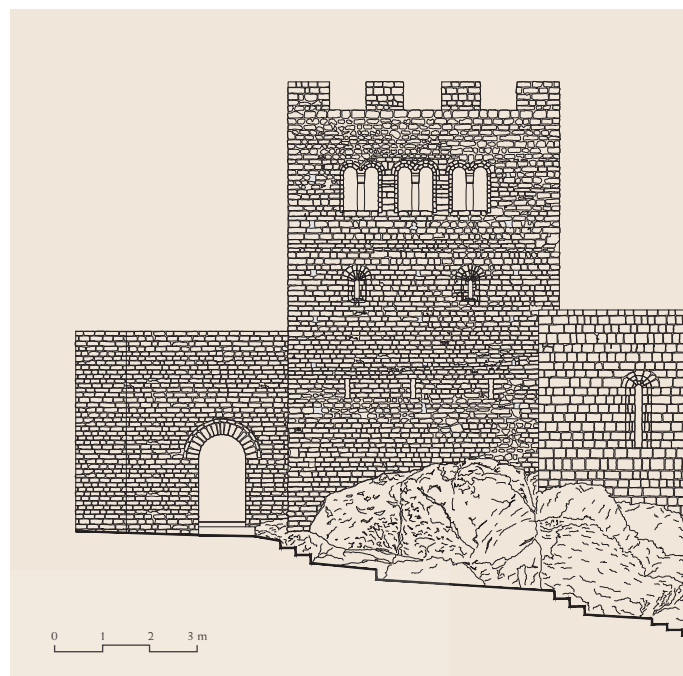
Alzado sur de la Torre de la Reina
