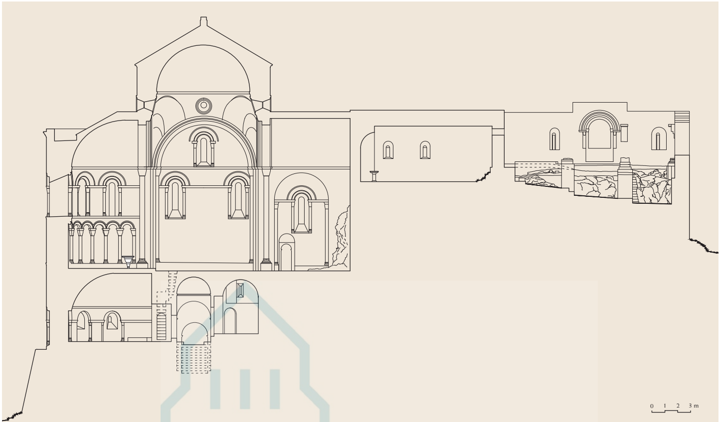
Sección longitudinal de la iglesia
