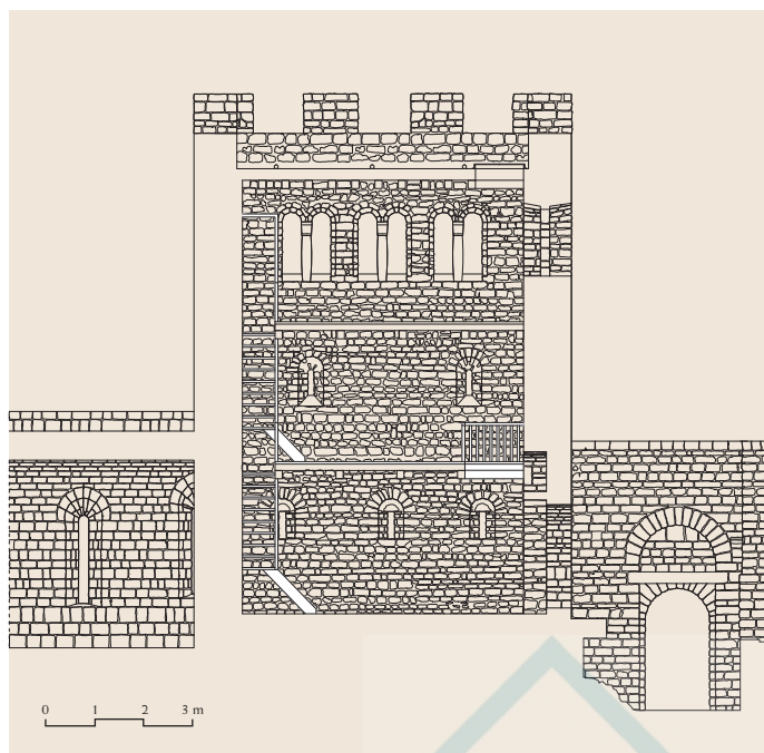
Sección longitudinal de la Torre de la Reina
