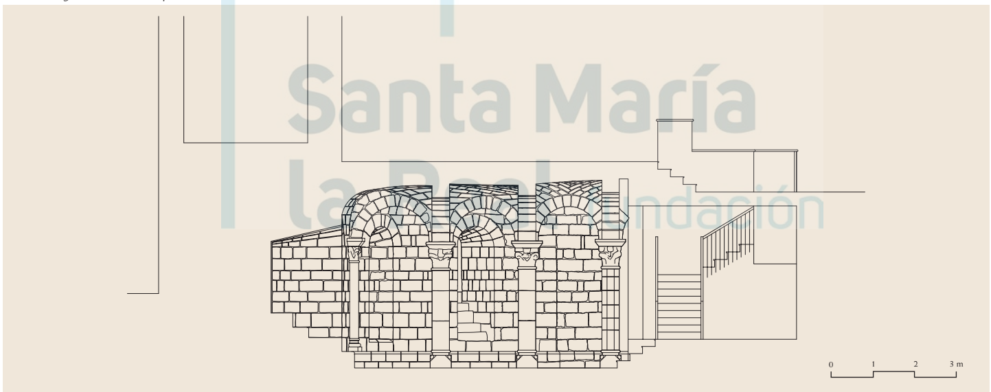
Sección longitudinal de la cripta
