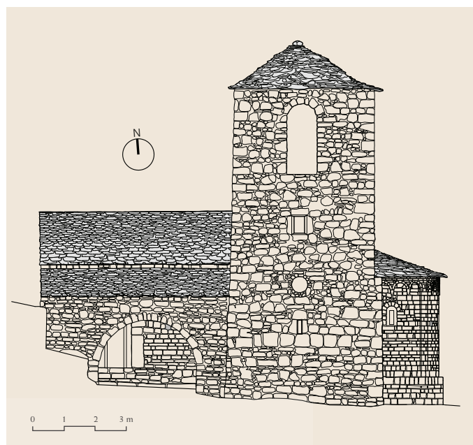
Alzado sur
