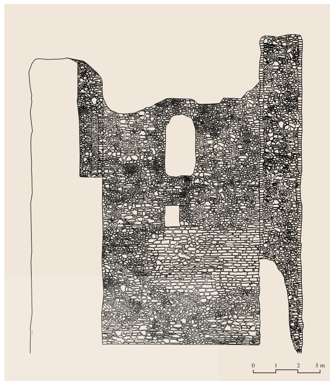
Sección transversal
