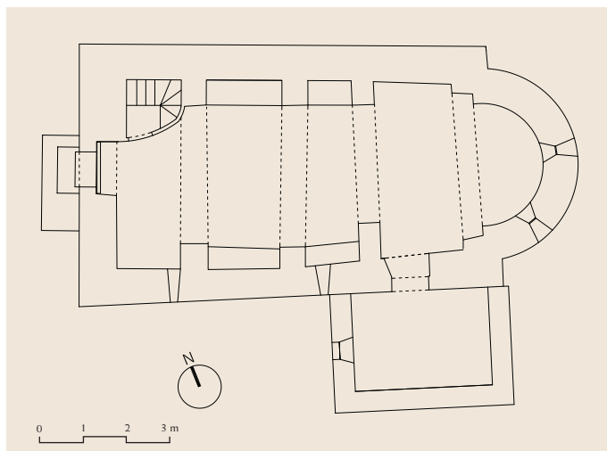
Planta
