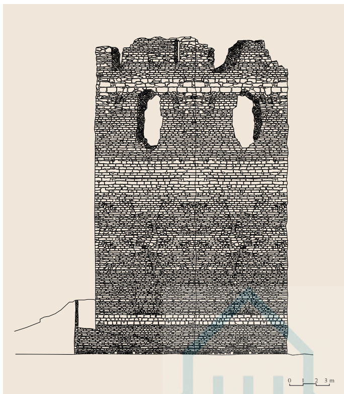
Alzado norte
