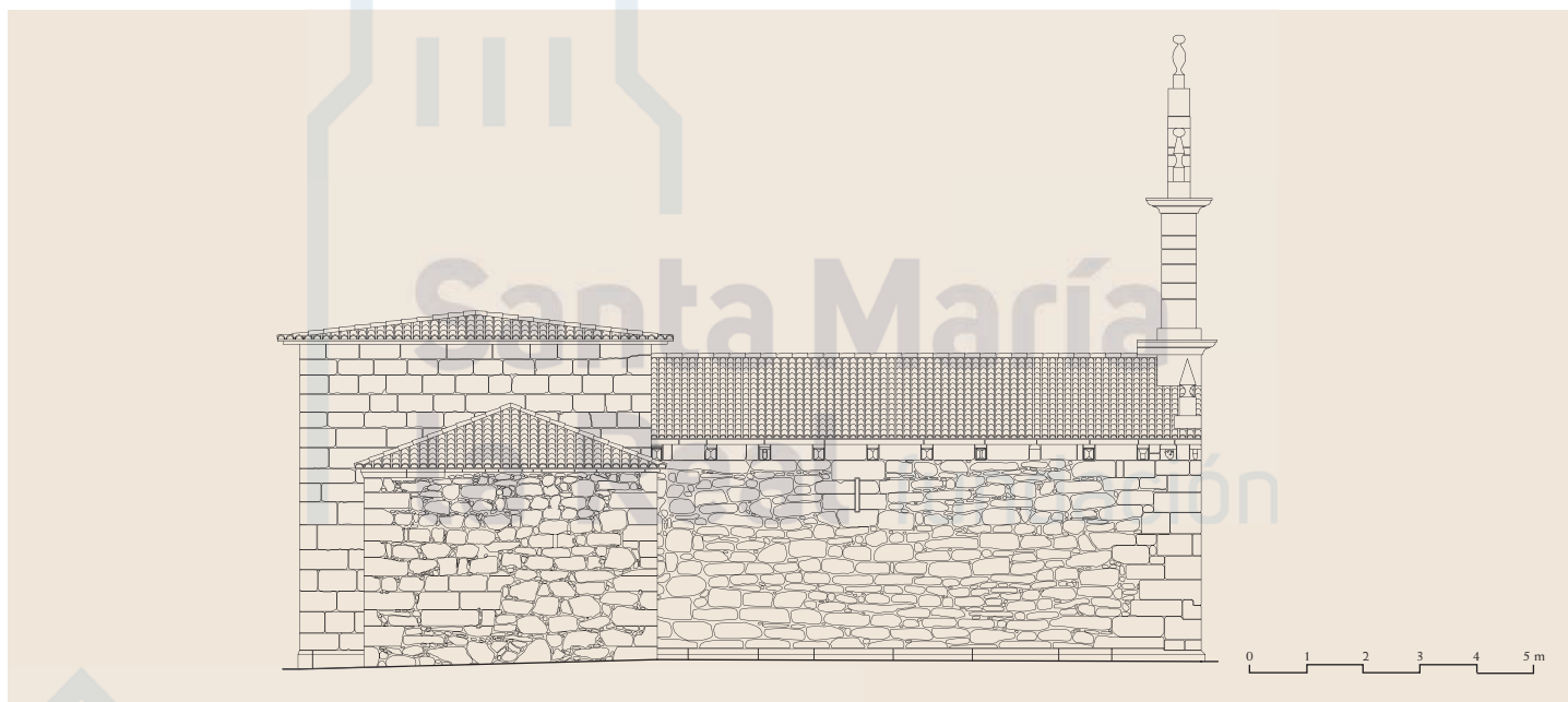
Alzado norte
