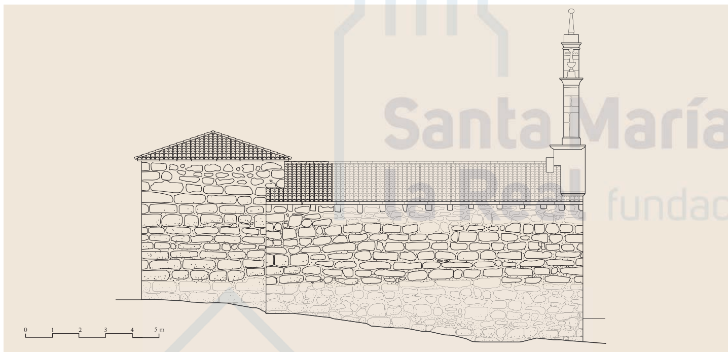
Alzado norte
