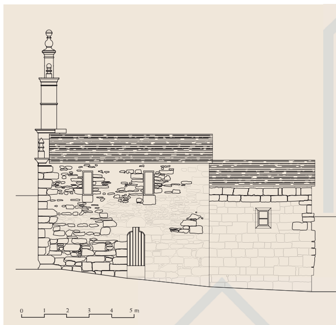
Alzado sur
