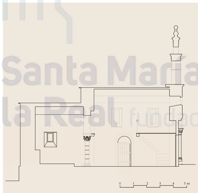
Sección longitudinal
