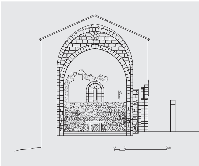
Secció transversal
