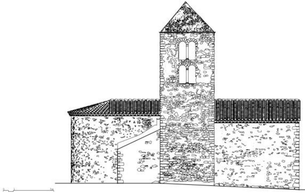
Alzado norte
