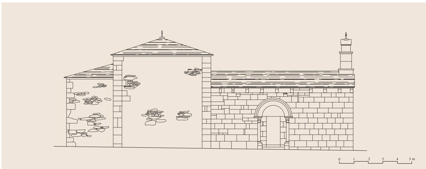
Alzado norte
