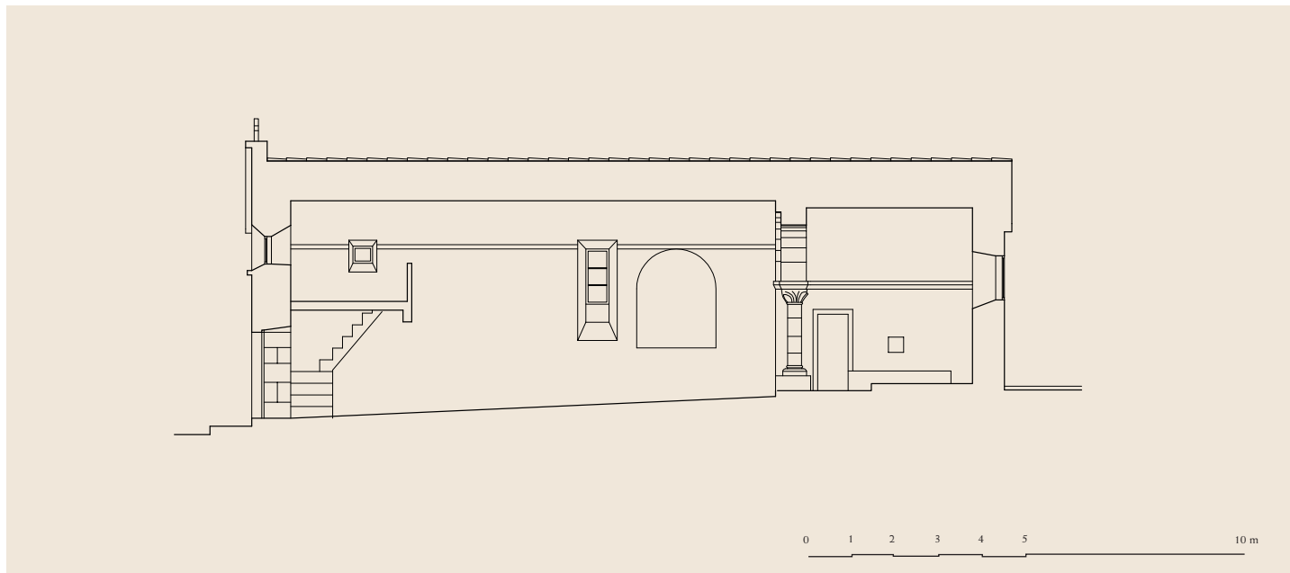
Sección longitudinal
