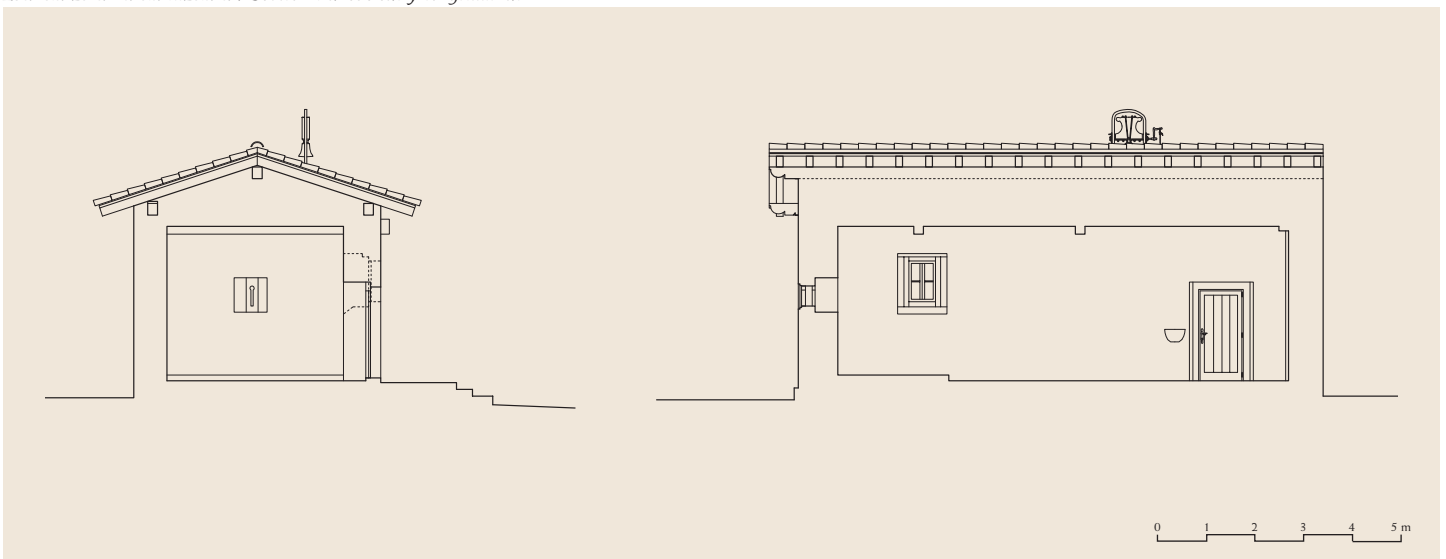
Ebaketa zebarka eta luzetara / Sección transversal y longitudinal
