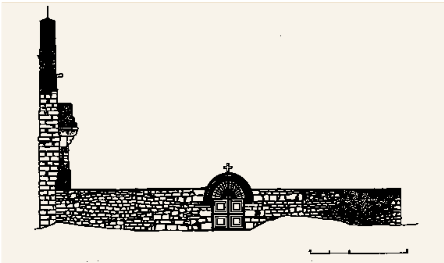
Alzado sur
