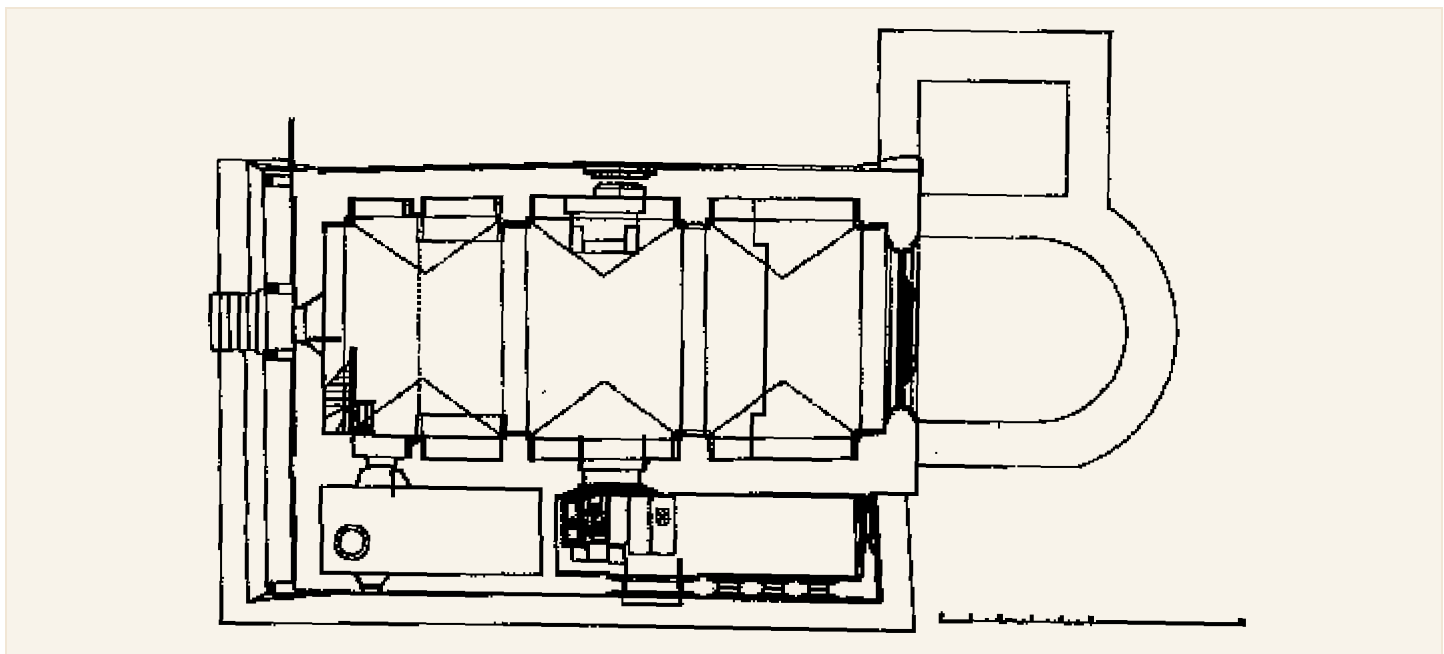
Planta (cabecera marcada en trazo fino, entonces caída después reconstruida)
