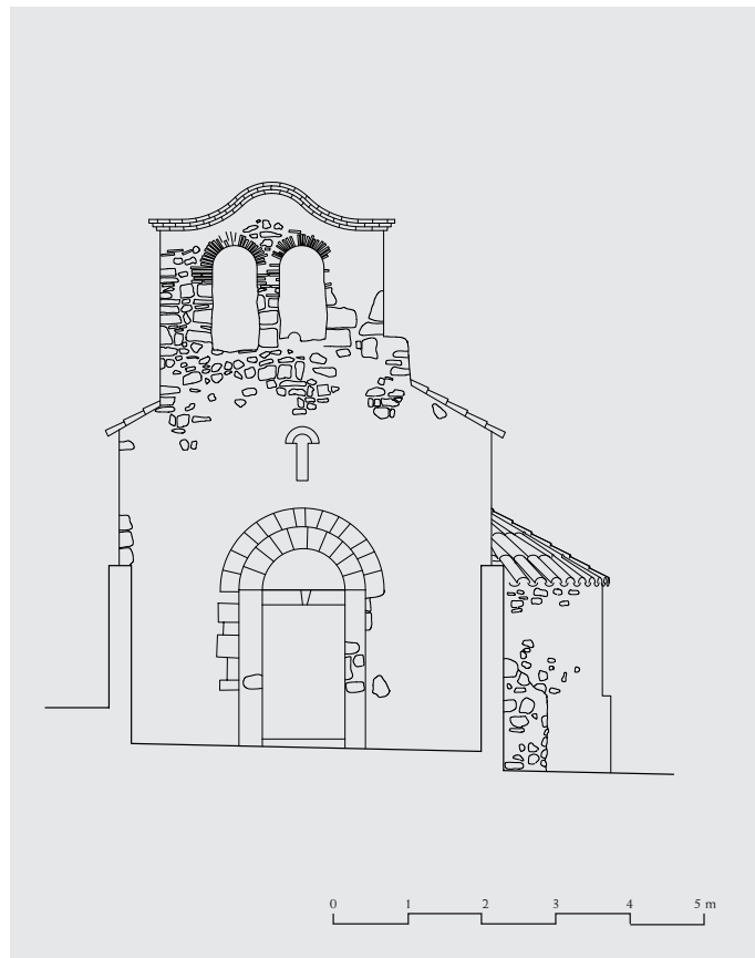
Alzado oeste
