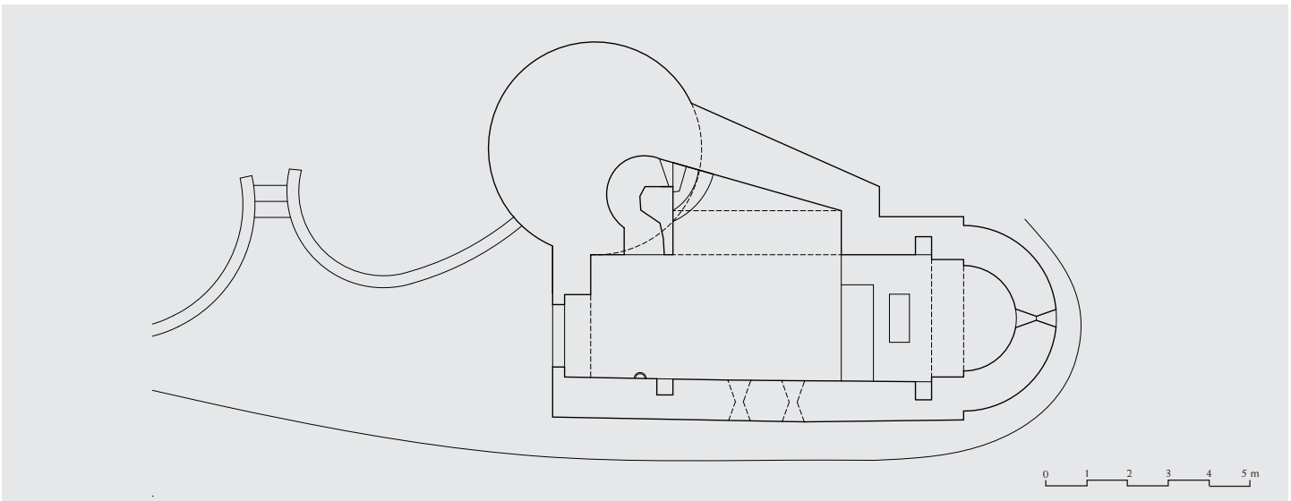
Planta
