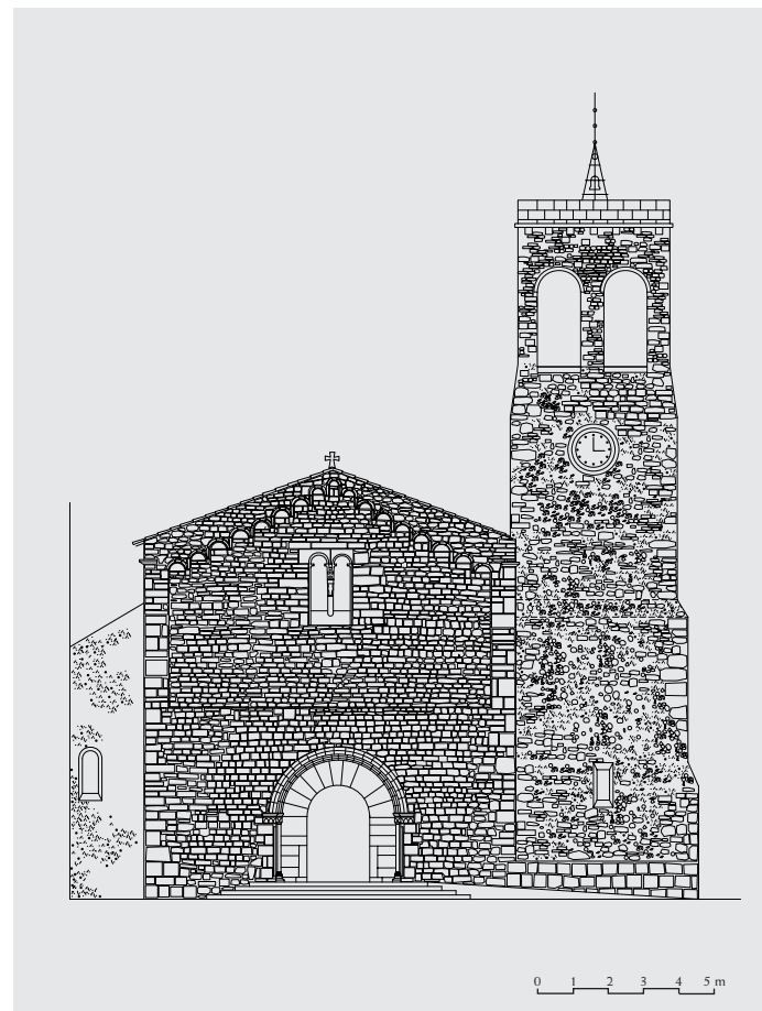
Alzado oeste
