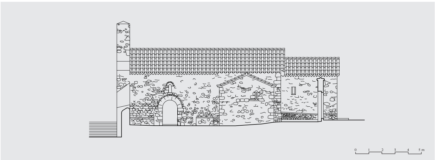
Alzado sur
