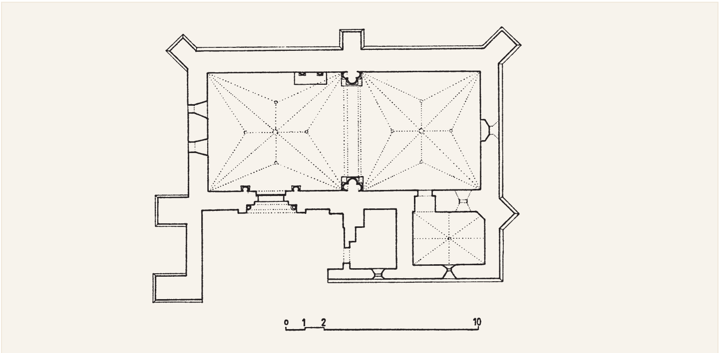
Planta, antes de la restauración
