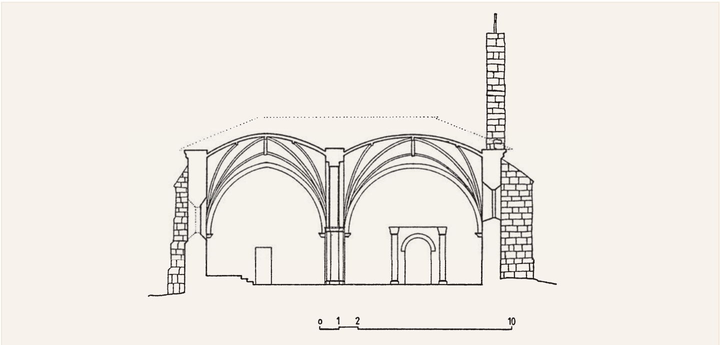
Sección longitudinal, antes de la restauración
