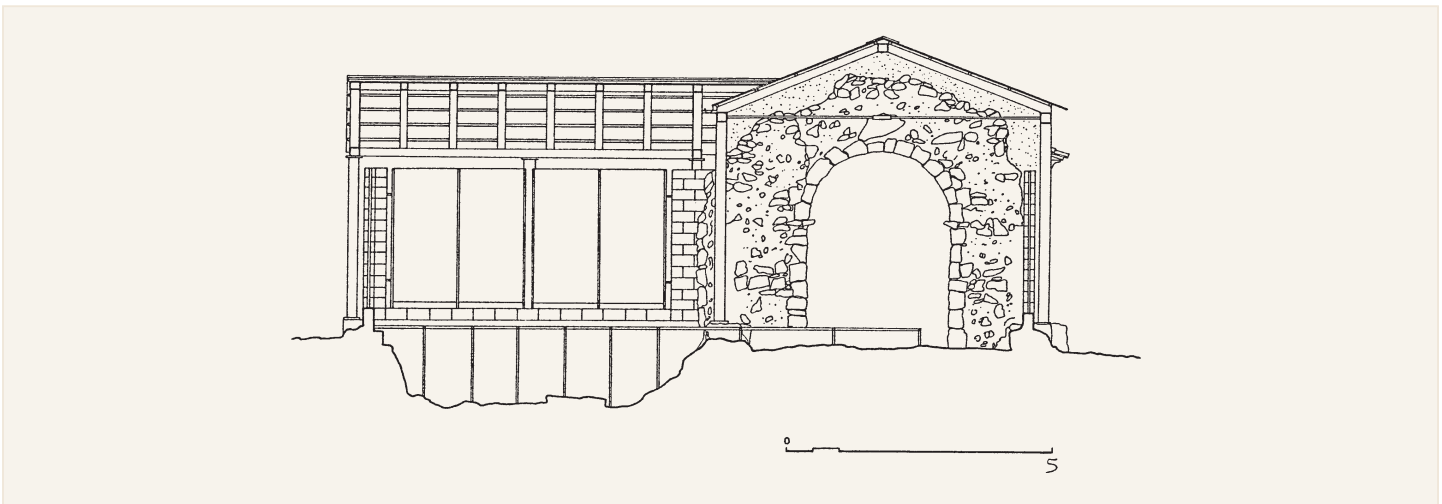
Sección transversal
