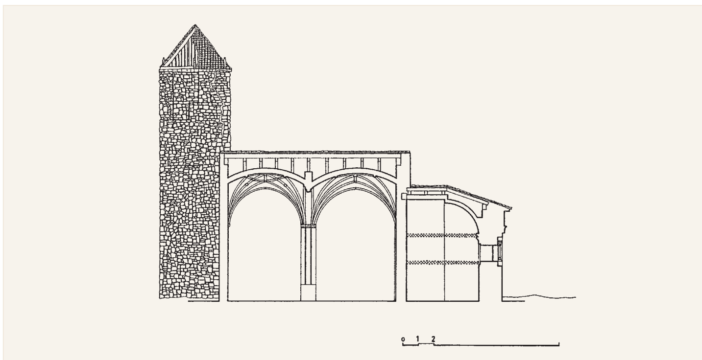
Sección longitudinal
