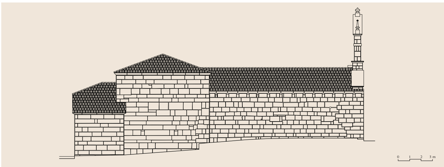
Alzado norte
