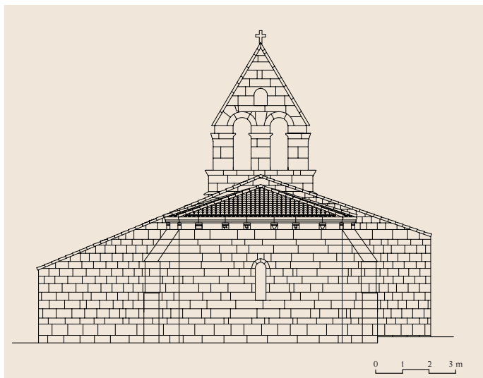
Alzado este
