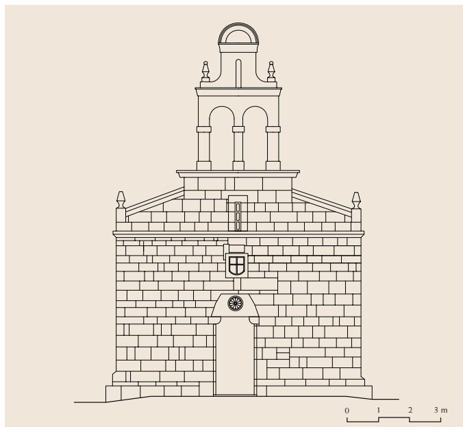
Alzado oeste
