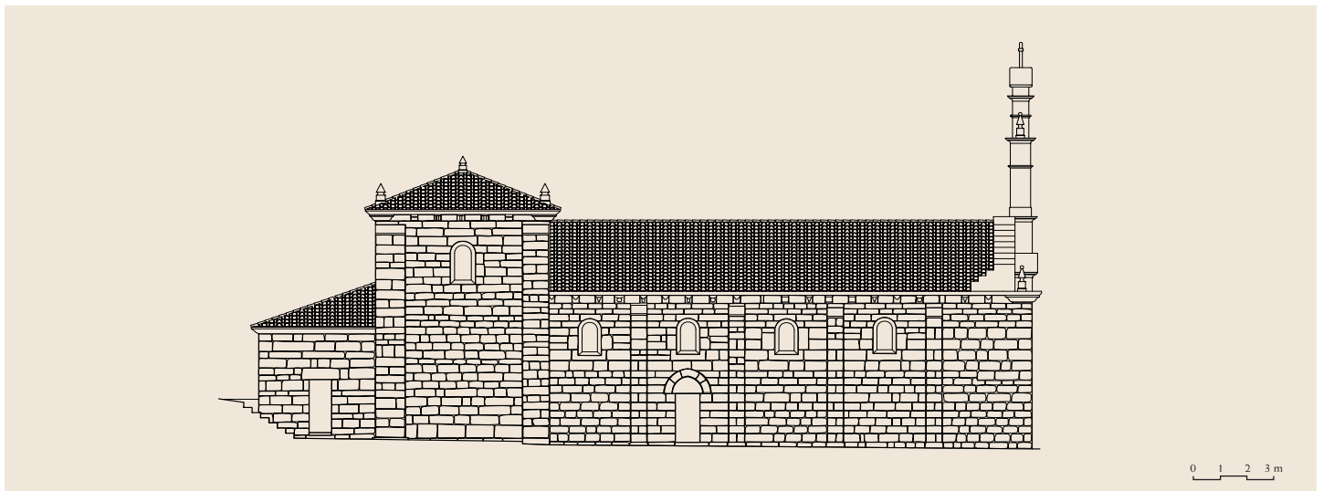
Alzado norte
