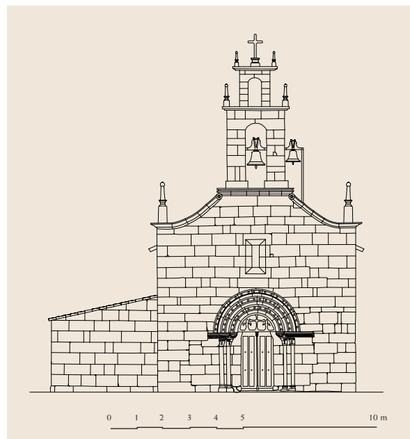
Alzado oeste
