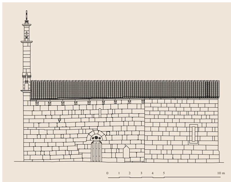
Alzado sur
