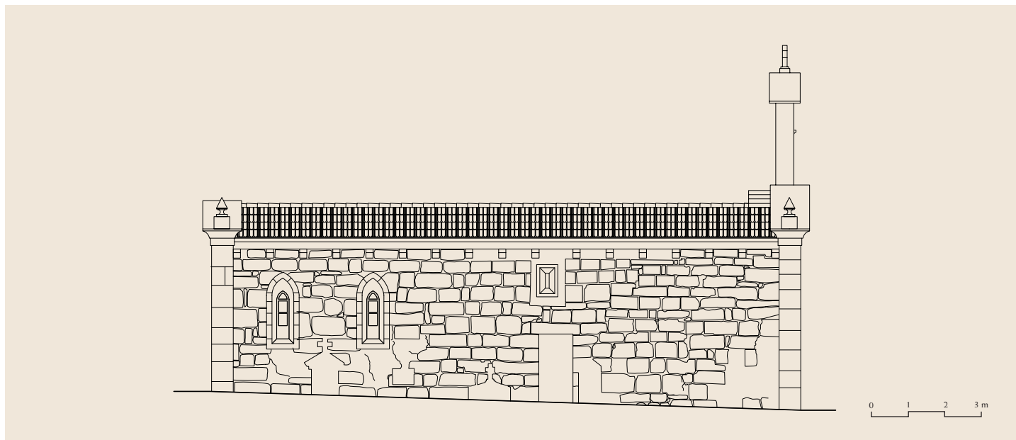
Alzado norte
