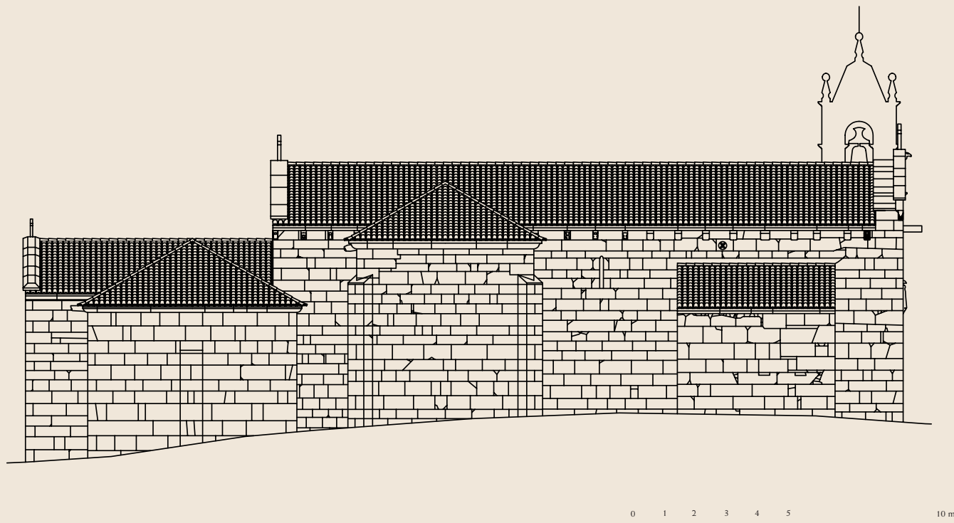
Alzado norte
