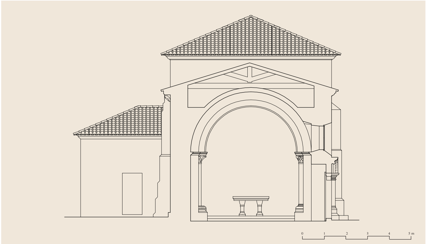
Sección transversal
