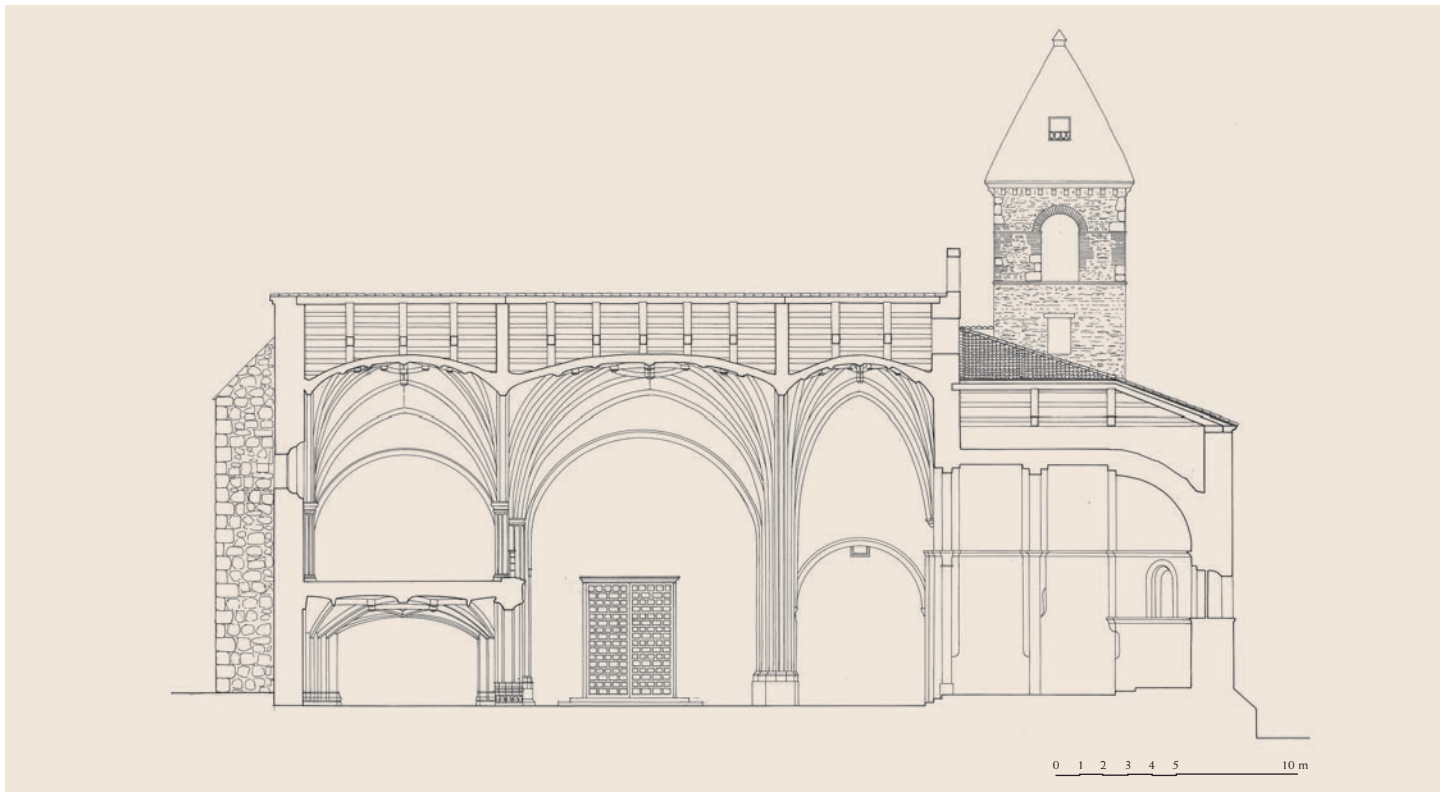
Sección longitudinal
