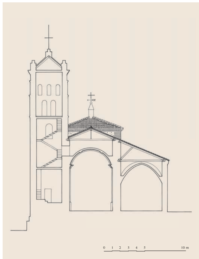
Sección transversal
