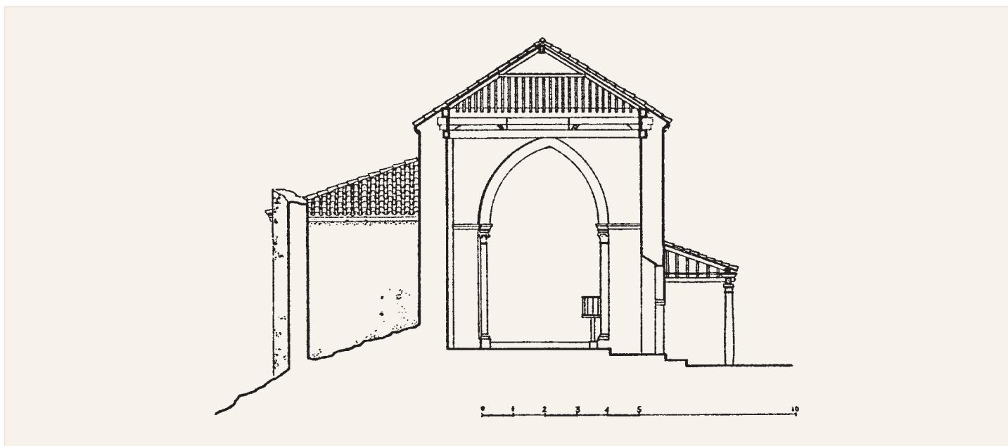
Sección transversal
