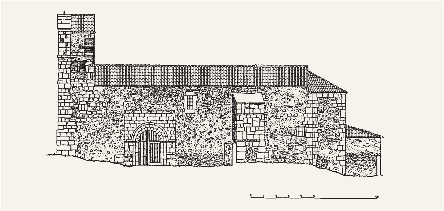
Alzado sur
