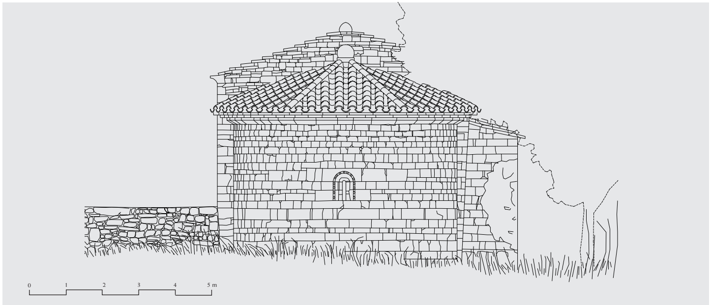
Alzado este
