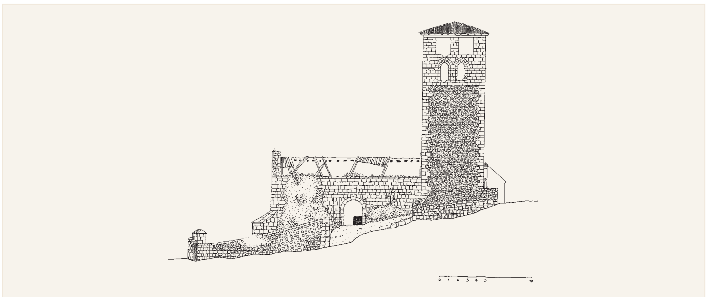
Alzado sur
