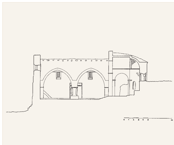
Sección longitudinal
