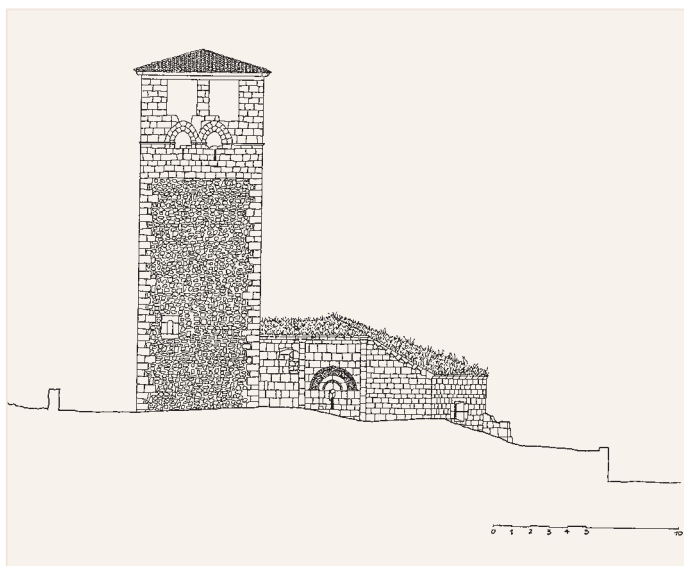
Alzado este
